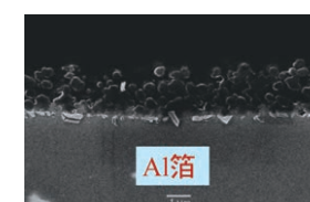
■トーヤルカーボ®の断面SEM像
