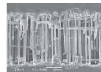
トーヤルパス®の断面の電子顕微鏡観察
